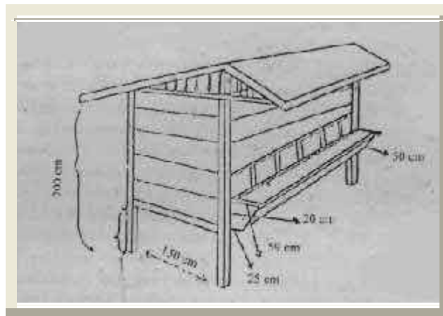
" Kontruksi Gambar Kandang Yang Ideal "
